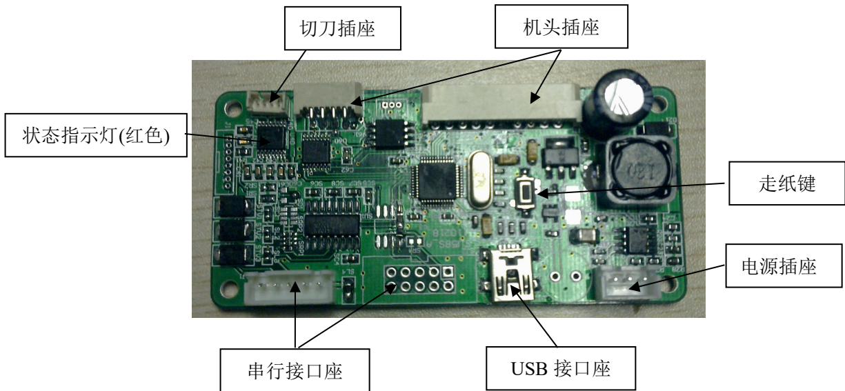
图 3-1 SP-EU58S 主控制板外观图
