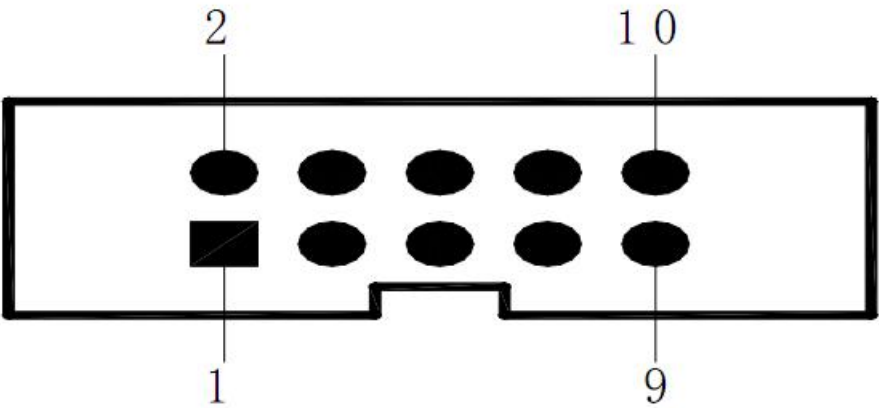
图 3-4 SP-EU58III IDC-10 型插座串行接口引脚序号定义
