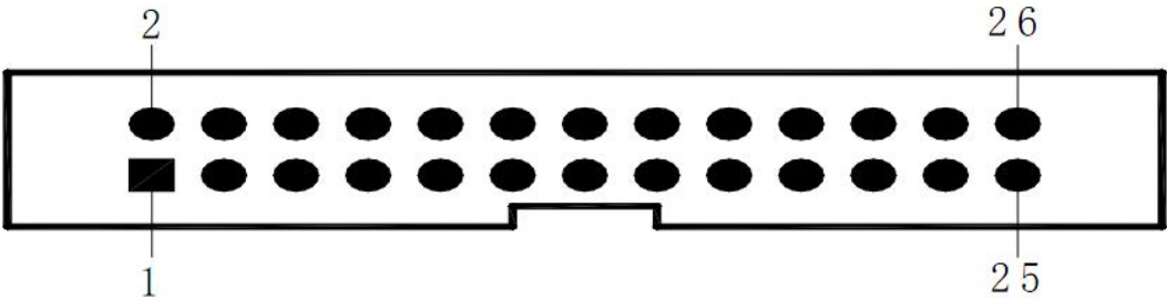
图 3-5 SP-EU58III 嵌入式打印单元并行接口插座引脚序号
