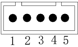
图 3-2 SP-EU58III 5PIN 单排串行接口插座引脚序号
