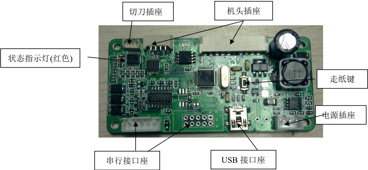
图 3-1 SP-EU58III 嵌入式打印单元主控制板外观图
