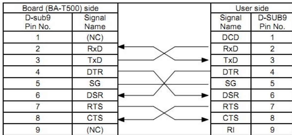
图 2-2 打印机串行接口与 PC 机串行接口连接示意图
