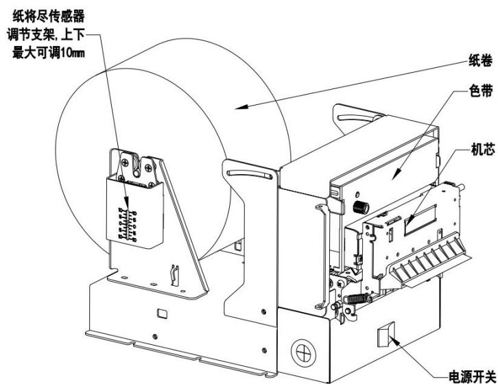
图2-1 打印单元组成
