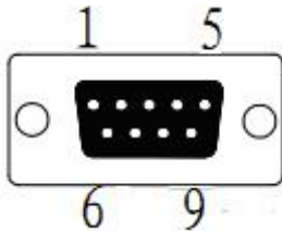
图2-2 串行接口插座引脚序号
