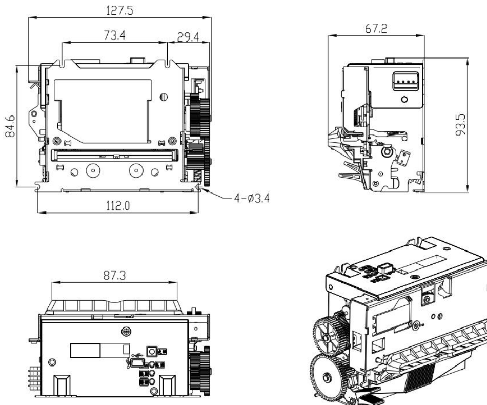
图 1-1 SP-EU803 嵌入式打印单元机型尺寸
