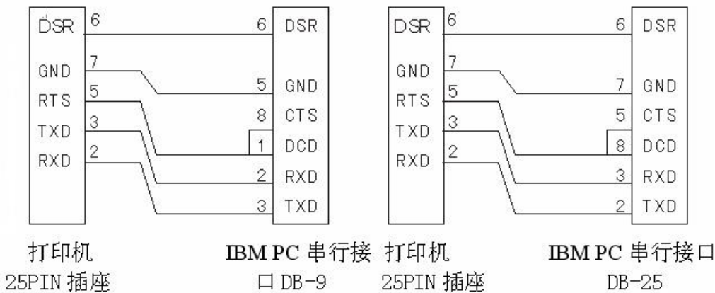
图 2-4 SP-POS586 打印机串行接口与 IBM PC 串行口连接示意图
