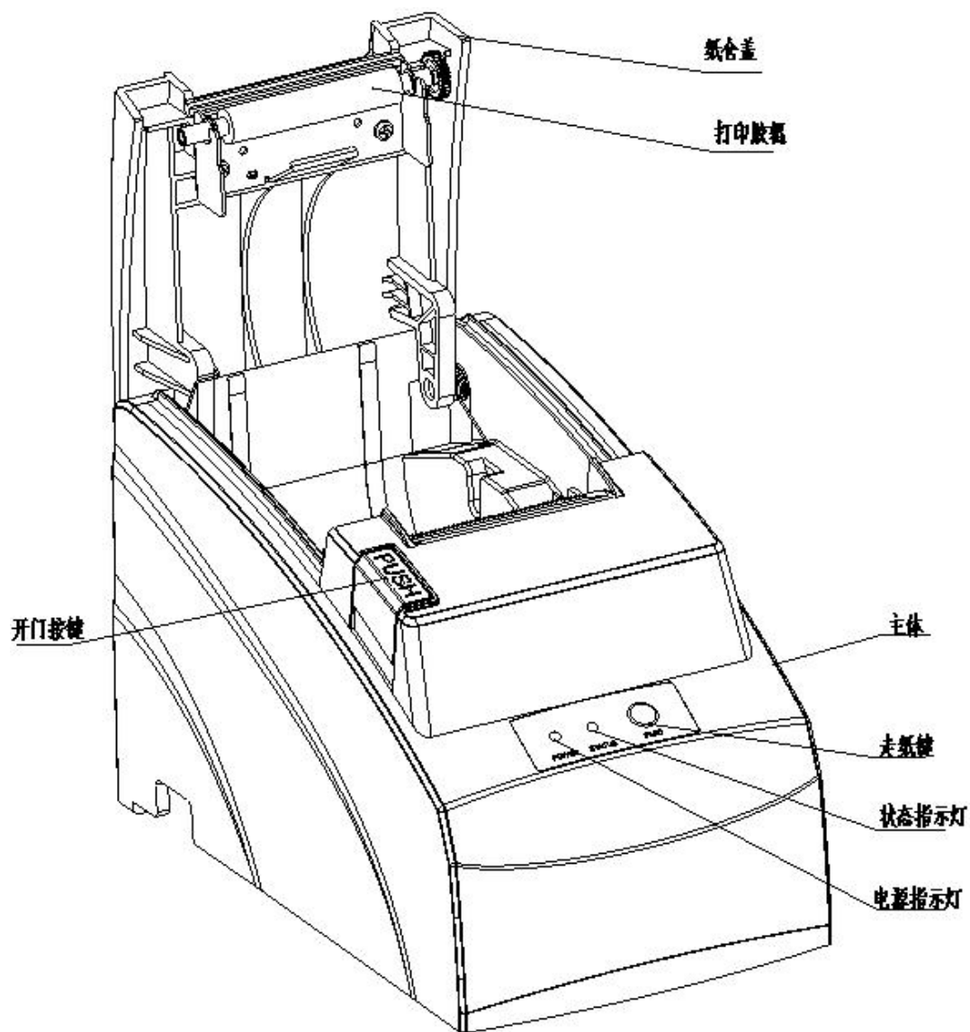
图 2-1 打印机外型
