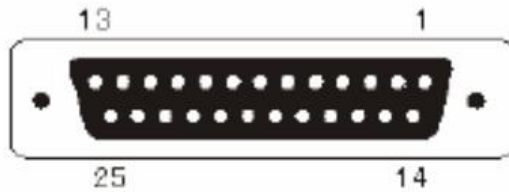
图 2-2 串行接口插座引脚序号
