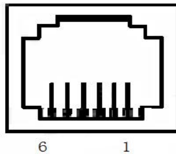
图 2-4 钱箱接口
