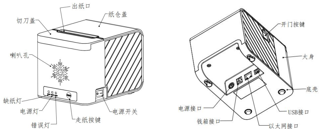
图 2-1 打印机各部分名称图
