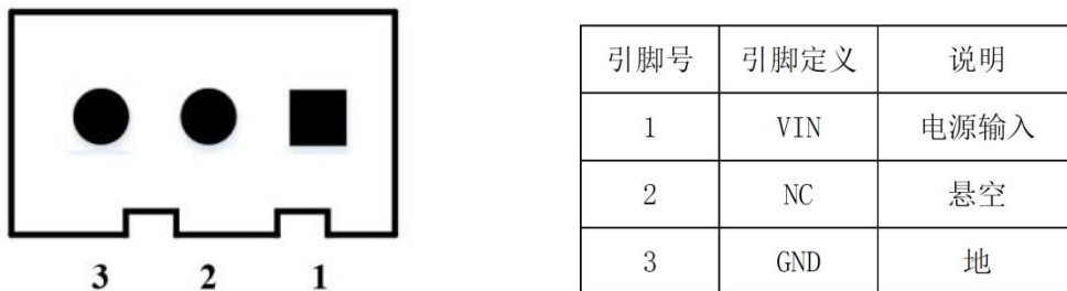
图 3-7 电源插座及引脚定义
