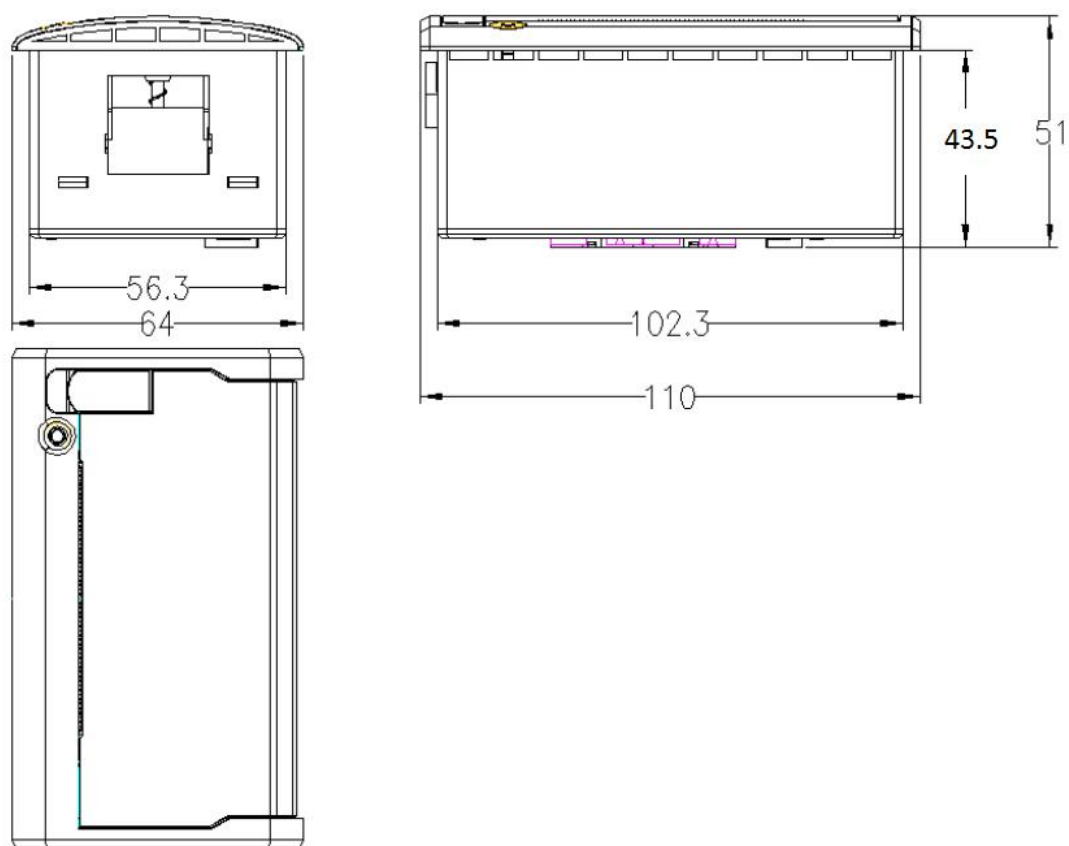
图 2-2 SP-RMD12 微型热敏打印机外形尺寸图
