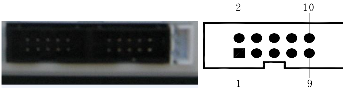
图3-1 串行接口IDC10针型插座引脚序号
