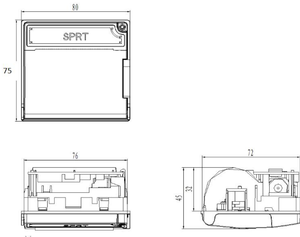
图 2-2 D15 外形尺寸图
