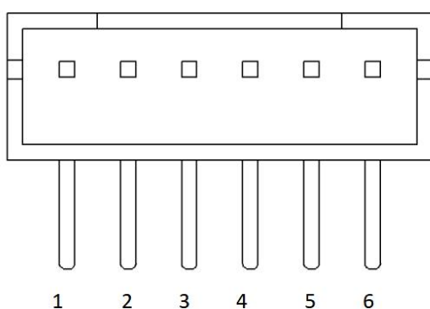
图 3-4 2mm 间距电源接口插座图
