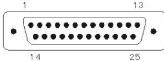
DB-25 并行接口插座引脚序号
