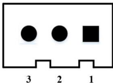
图 3-4 电源接口插座图
