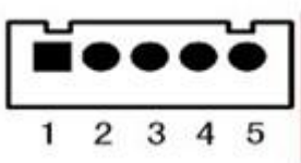
图3—2 5PIN单排串行接口插座引脚序号
