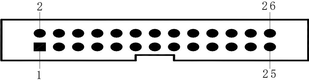
图3-3 并行接口插座引脚序号
