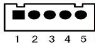
PDK-5单排串行接口插座引脚序号
