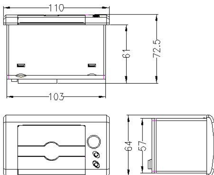
图 2-2 SP-RMDI11D 机型图
