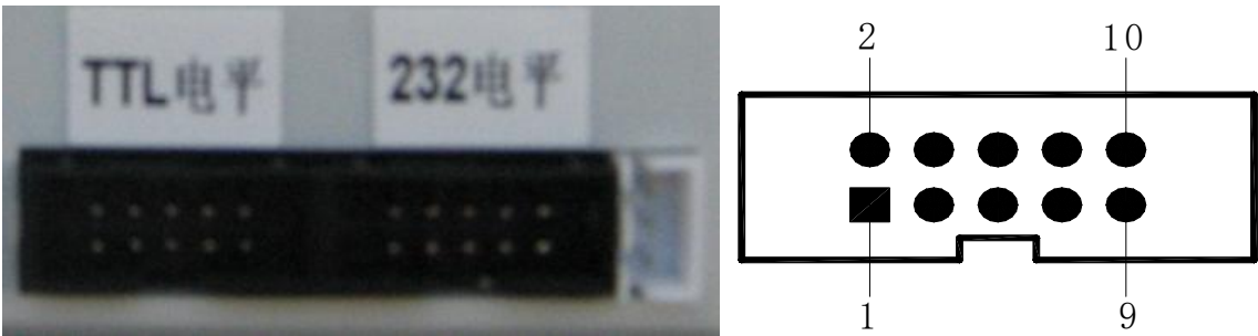
图3—1 串行接口IDC10针型插座引脚序号
