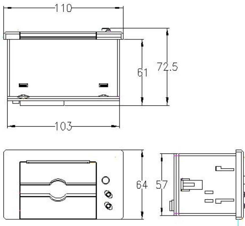
图 2—3 SP-RMD1VD 机型图
