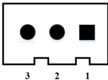
图 3-4 电源接口插座图
