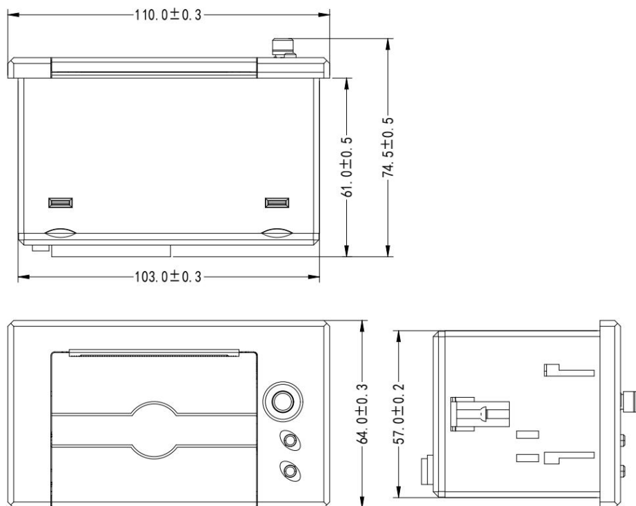
图 2—3 SP-RMD1VD 机型图
