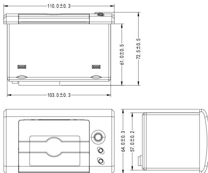
图 2-2 SP-RMDIIIID 机型图
