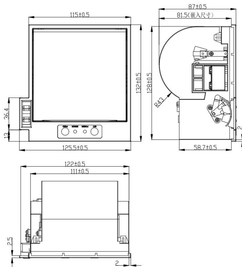
图 1-1 RME4 产品外形尺寸图
