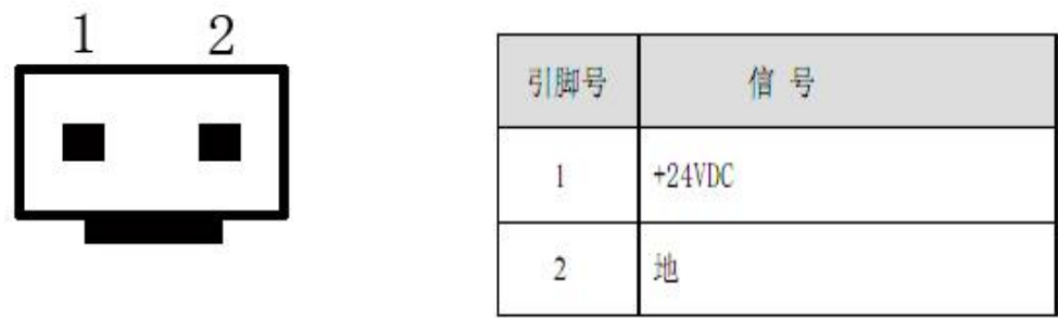
图 2-6 电源插座及引脚定义
